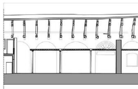
LONG SECTION B-B'
